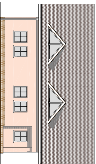
Z FASADA
