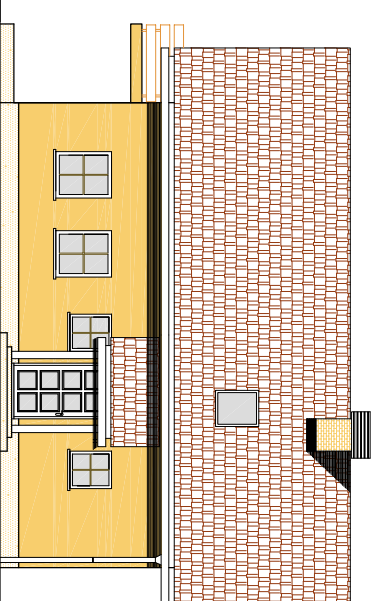
S FASADA
