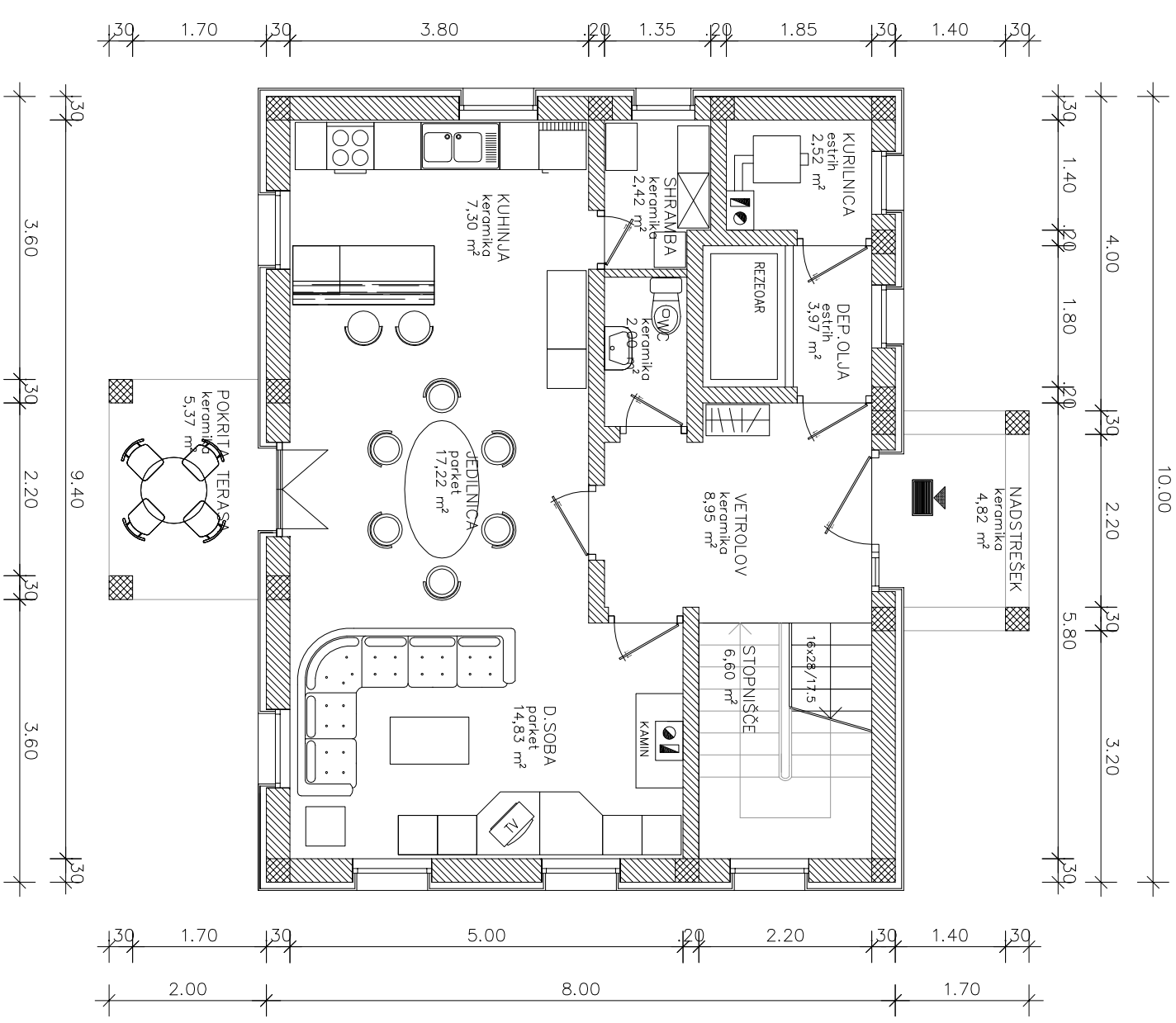
TLORIS PRITLIČJA
