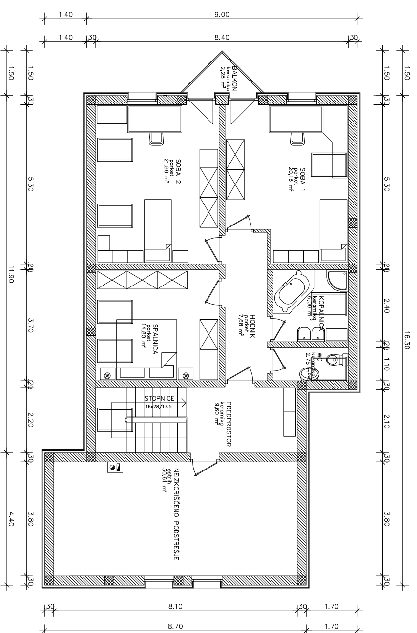
TLORIS MANSARDE
