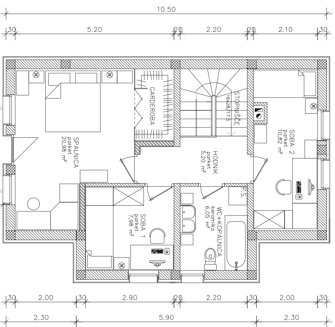
TLORIS MANSARDE
