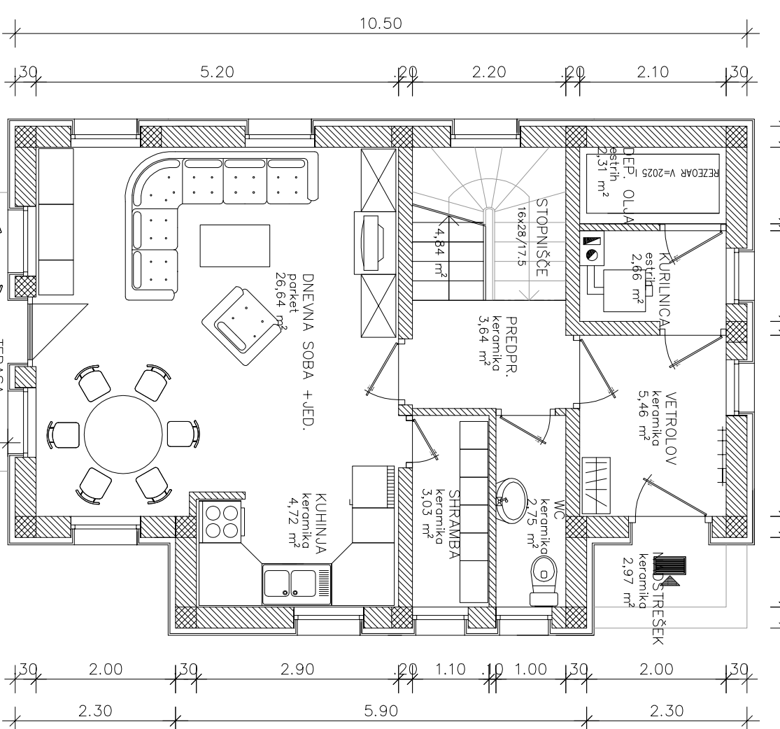
TLORIS PRITLIČJA
