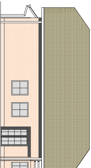
JZ FASADA
