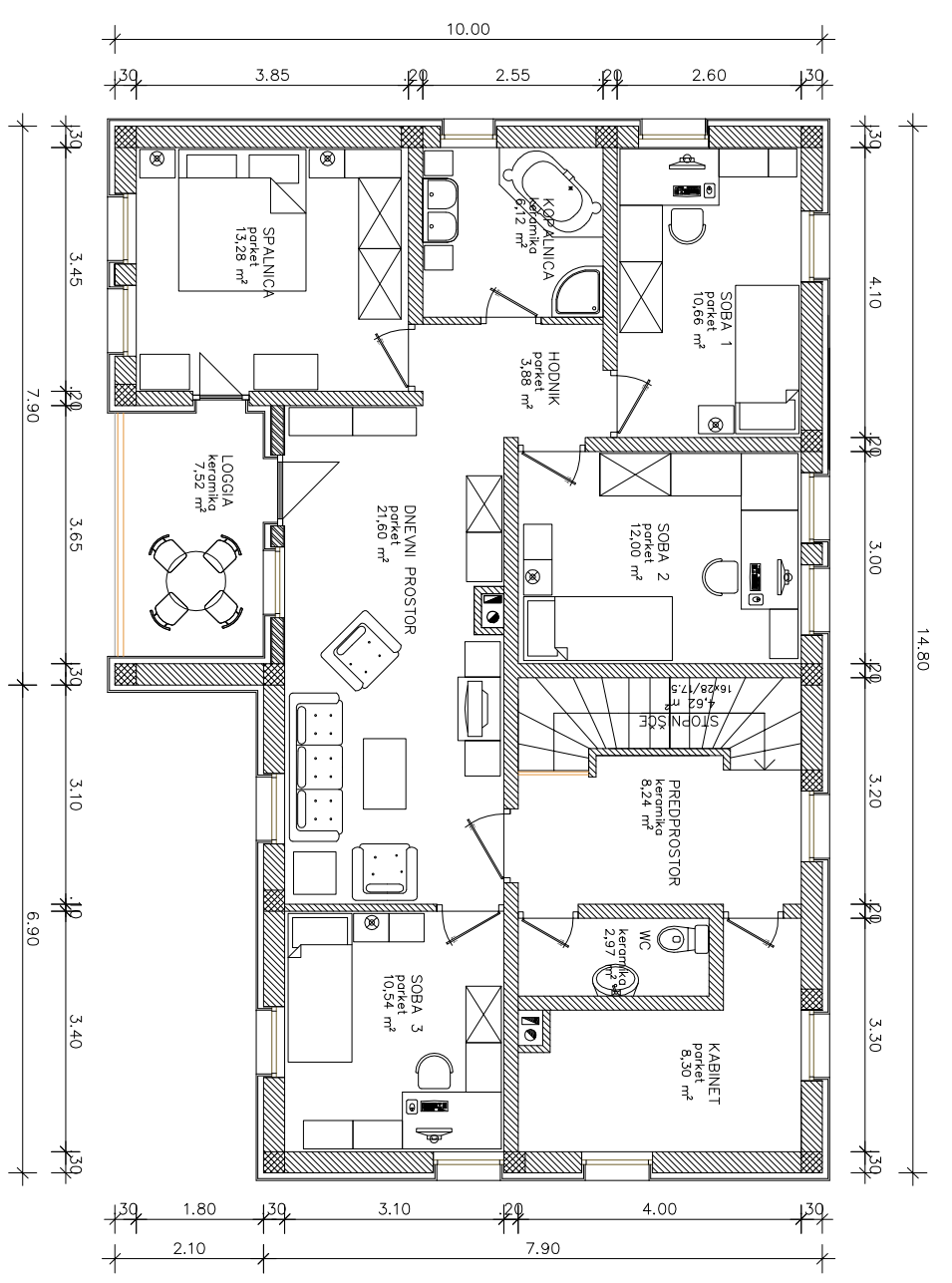
TLORIS MANSARDE
