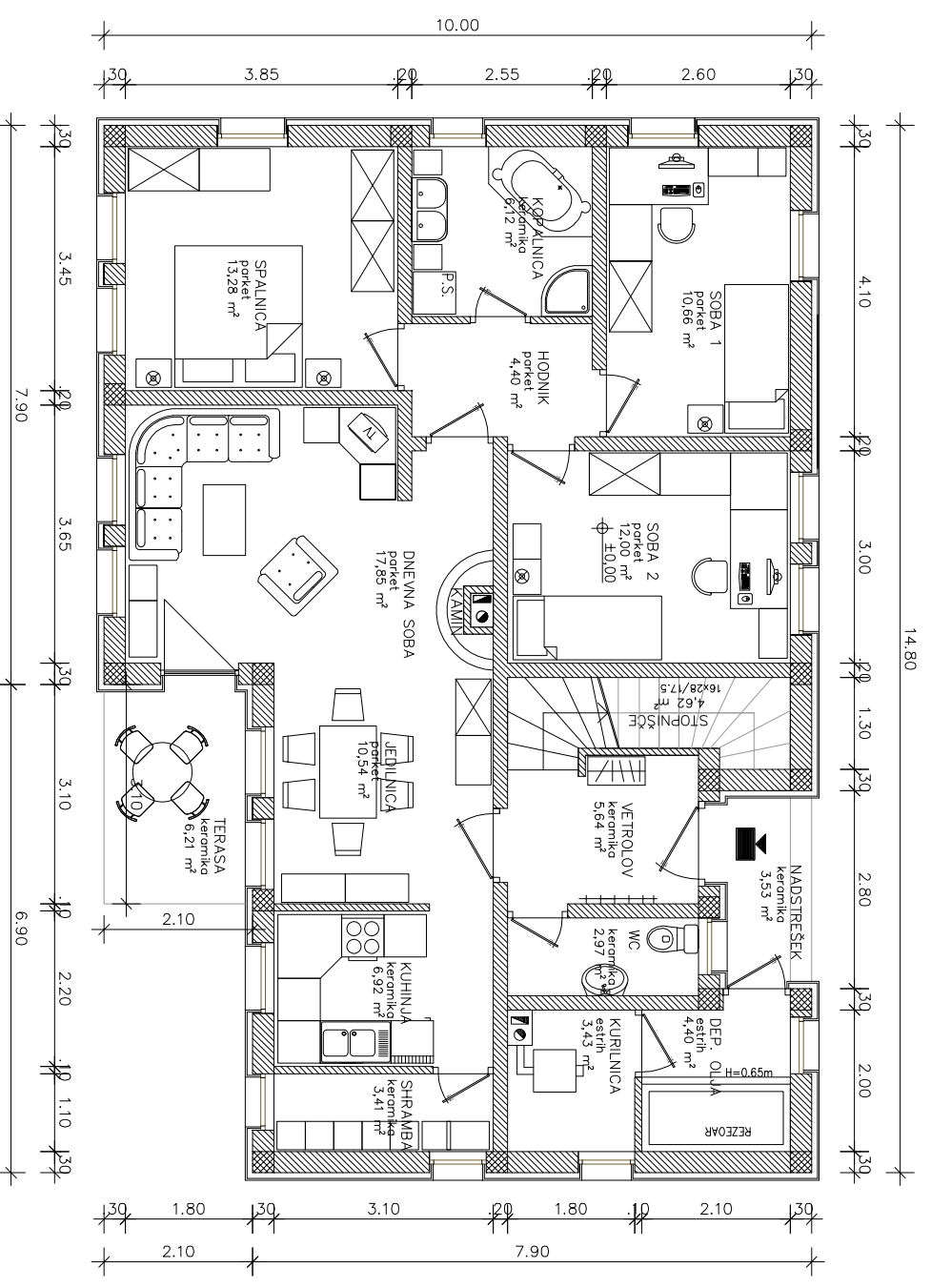
TLORIS PRITLIČJA
