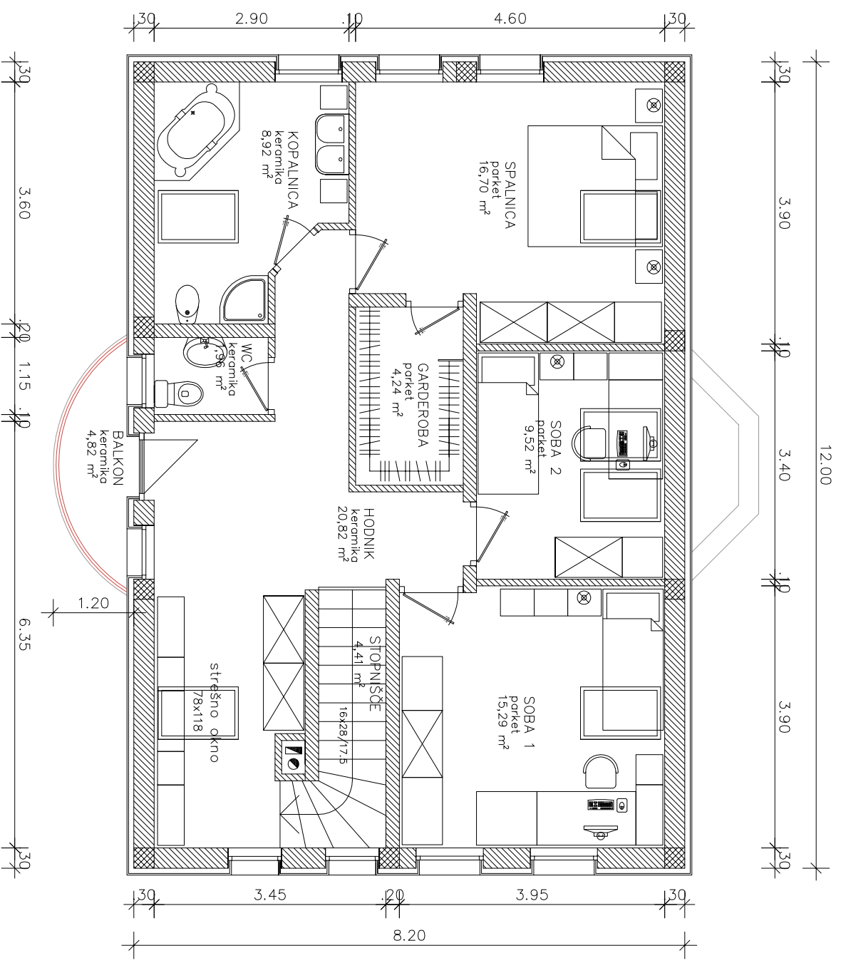
TLORIS MANSARDE
