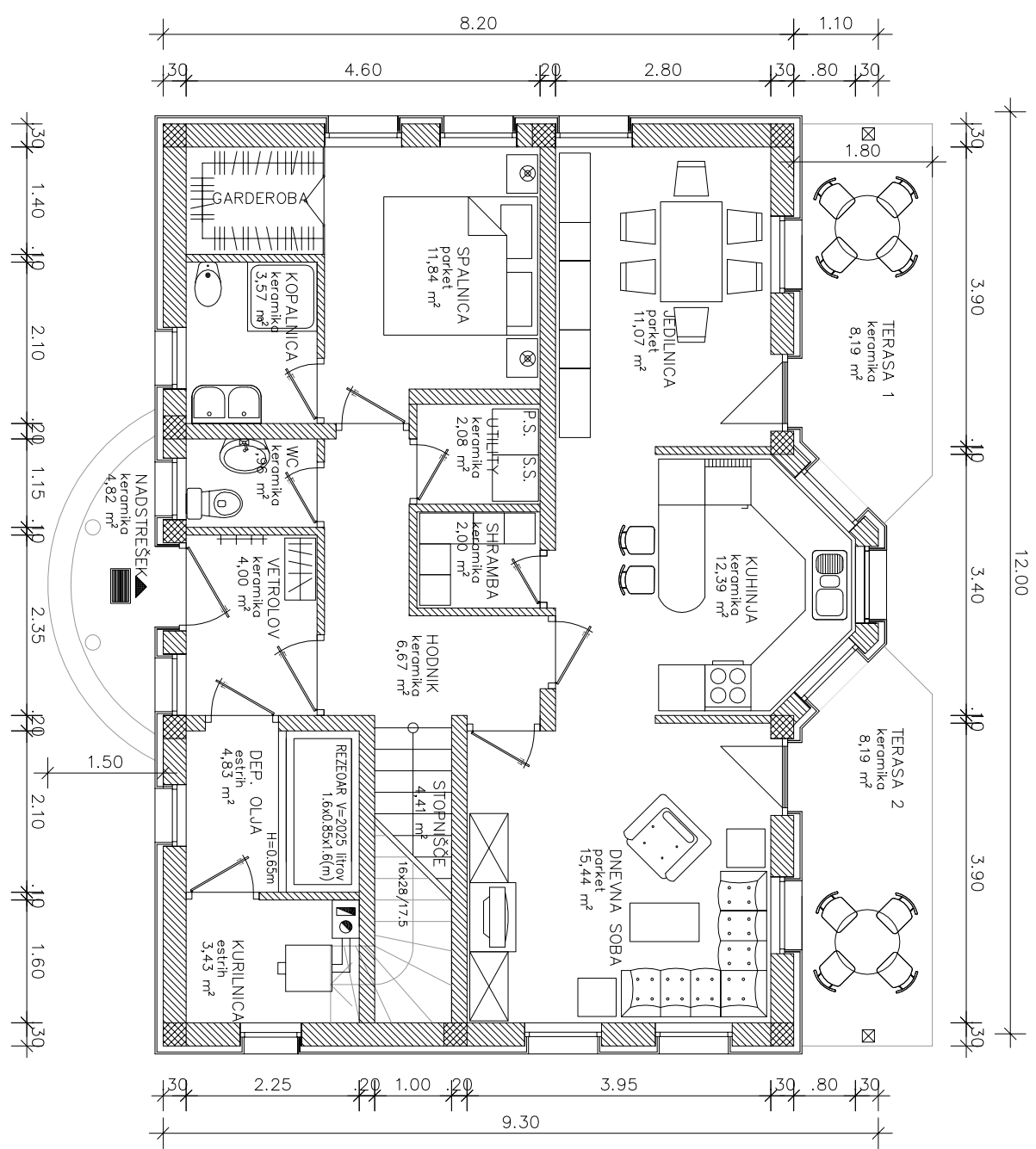
TLORIS PRITLIČJA
