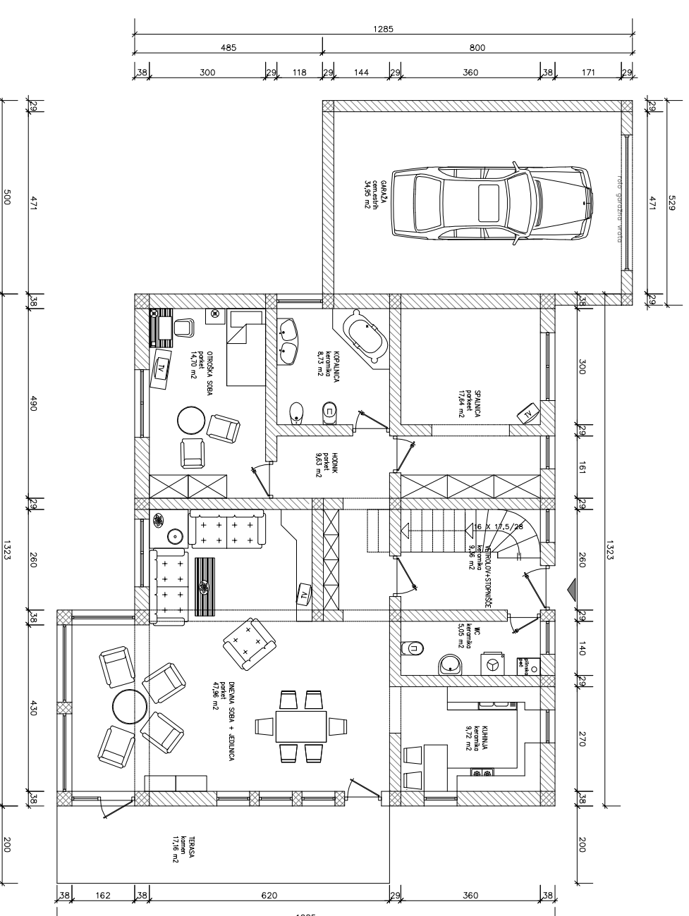
FLORIS PRITLIČJA
