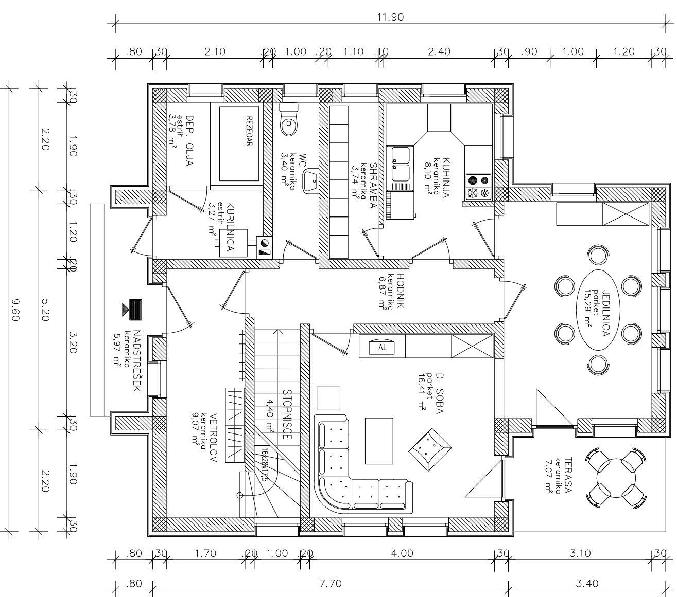
TLORIS PRITLIČJA
