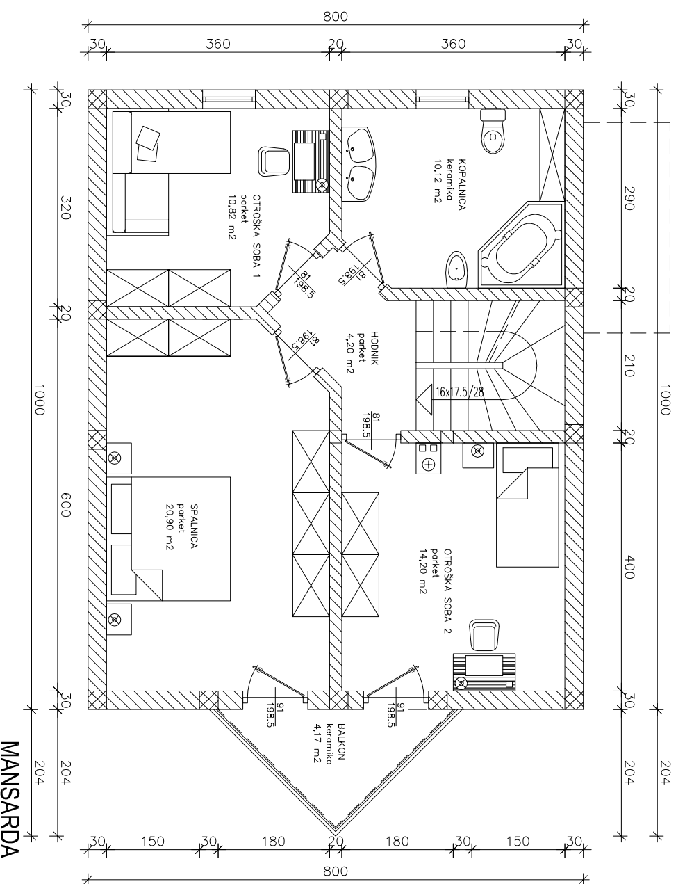
PRITLIČJE
