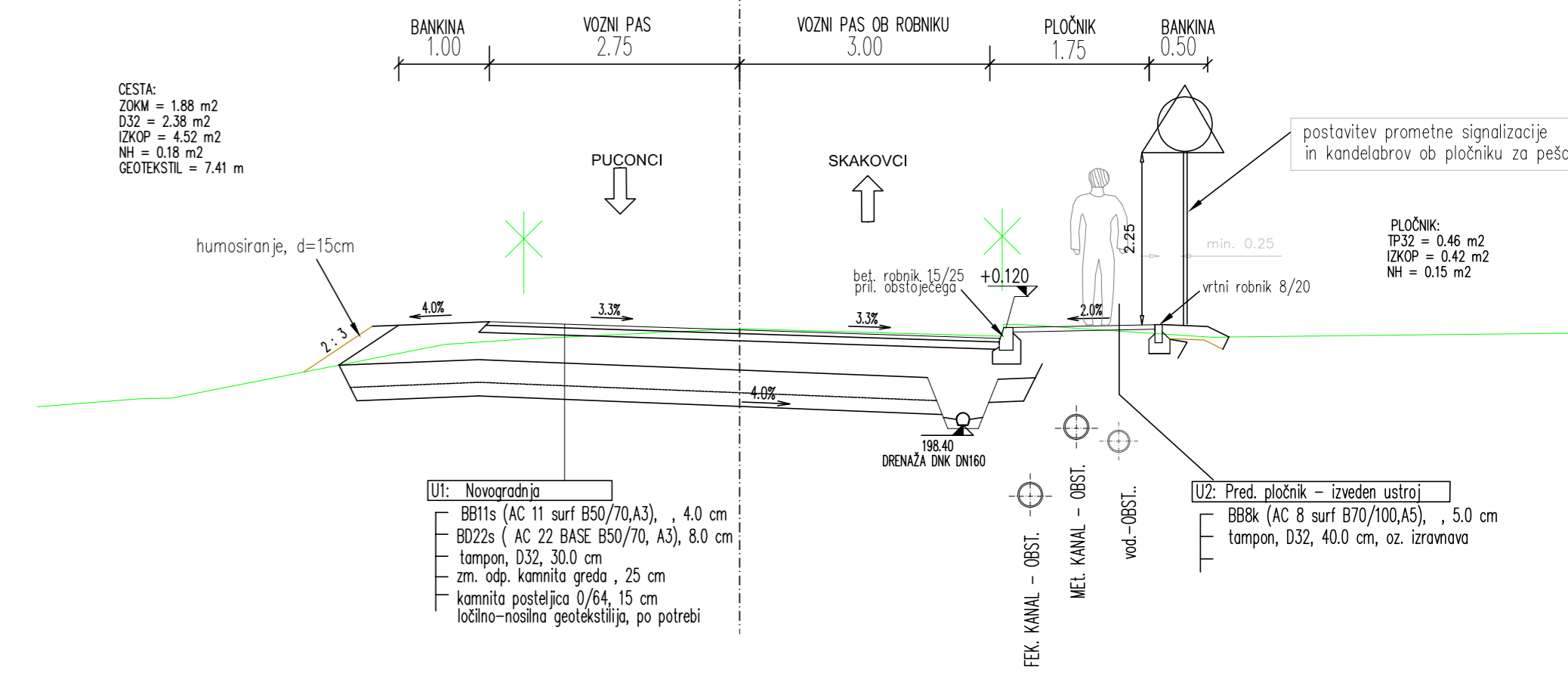
Karakteristični prerez R3-715/5645 v naselju od km 5+180 do km 5+953
